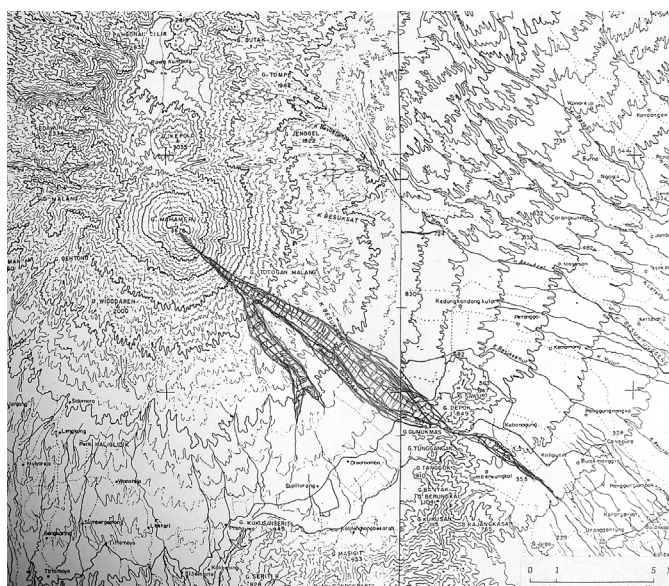
ブスック・コボカンから流れ出た火山砕屑流とラハールの流域(推定)
