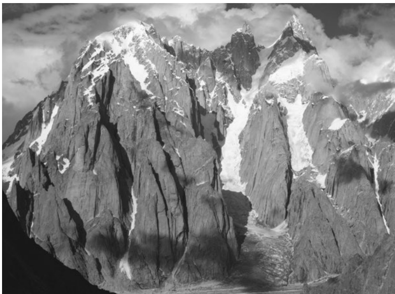
この写真では分かりづらいが、パダルピーク山頂から K7西峰までは3 km近い複雑なリッジが続く
